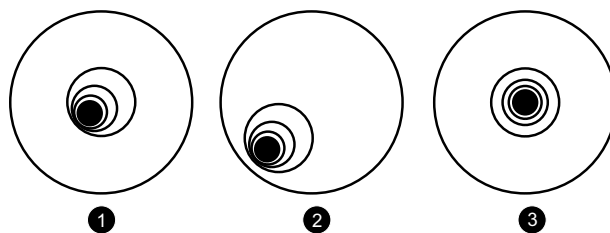
Расфокусированные изображения звезды. Не выровненные - 1,2, выровненное - 3
